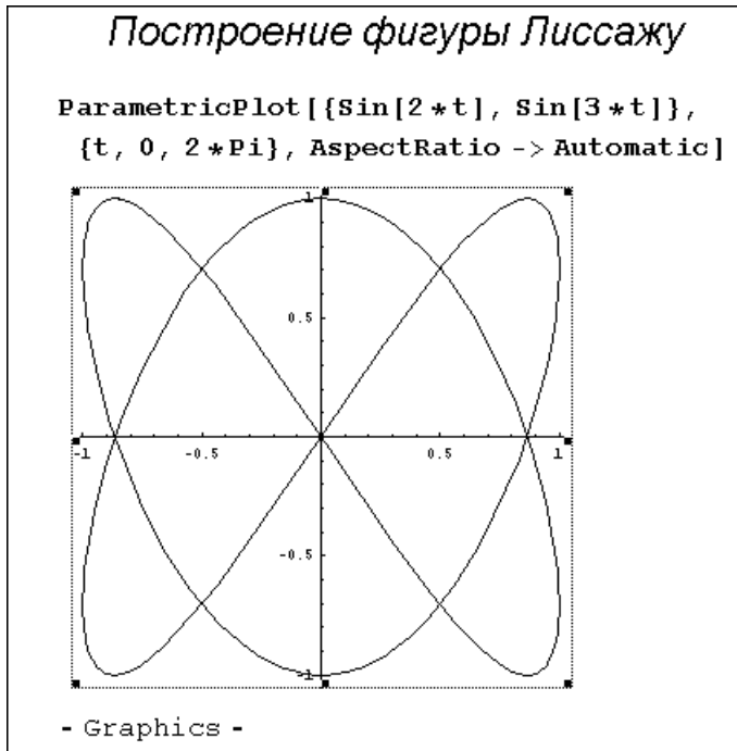
Рис. 8.12. Построение фигуры Лиссажу
