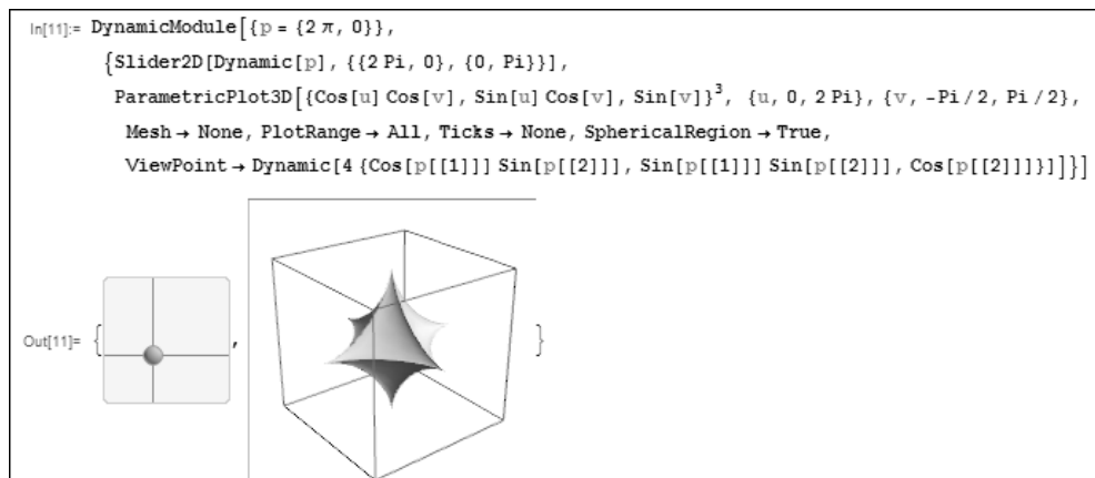
Рис. 8.54. Пример, иллюстрирующий вращение трехмерной фигуры в пространстве с помощью двухкоординатного слайдера
