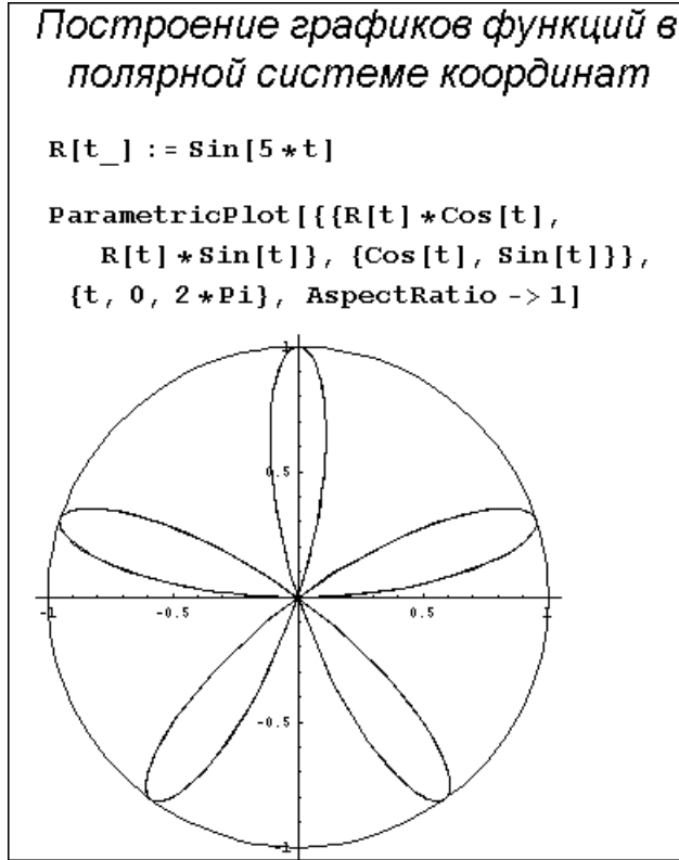
Рис. 8.14. Построение графика функции в полярной системе координат
