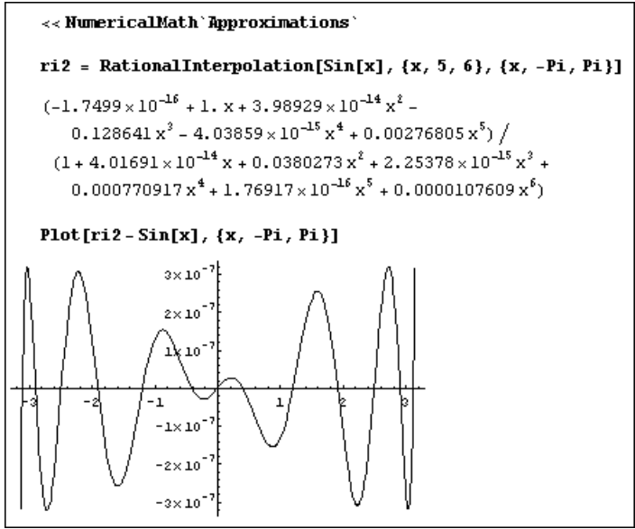
Рис. 6.14. Пример рациональной аппроксимации синусоидальной функции
